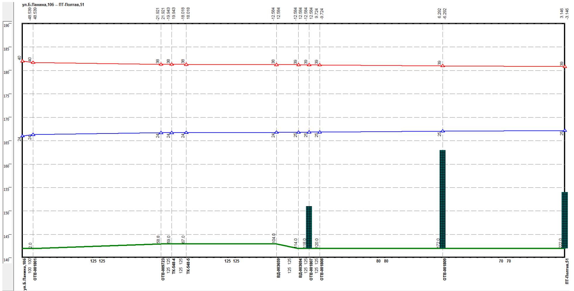
Рисунок Ошибка! Текст указанного стиля в документе отсутствует..178 –Результат гидравлического расчета - график гидравлических режимов по пути теплоносителя от котельной Бориса Панина, 10-б до ПТ-Полтав,51
