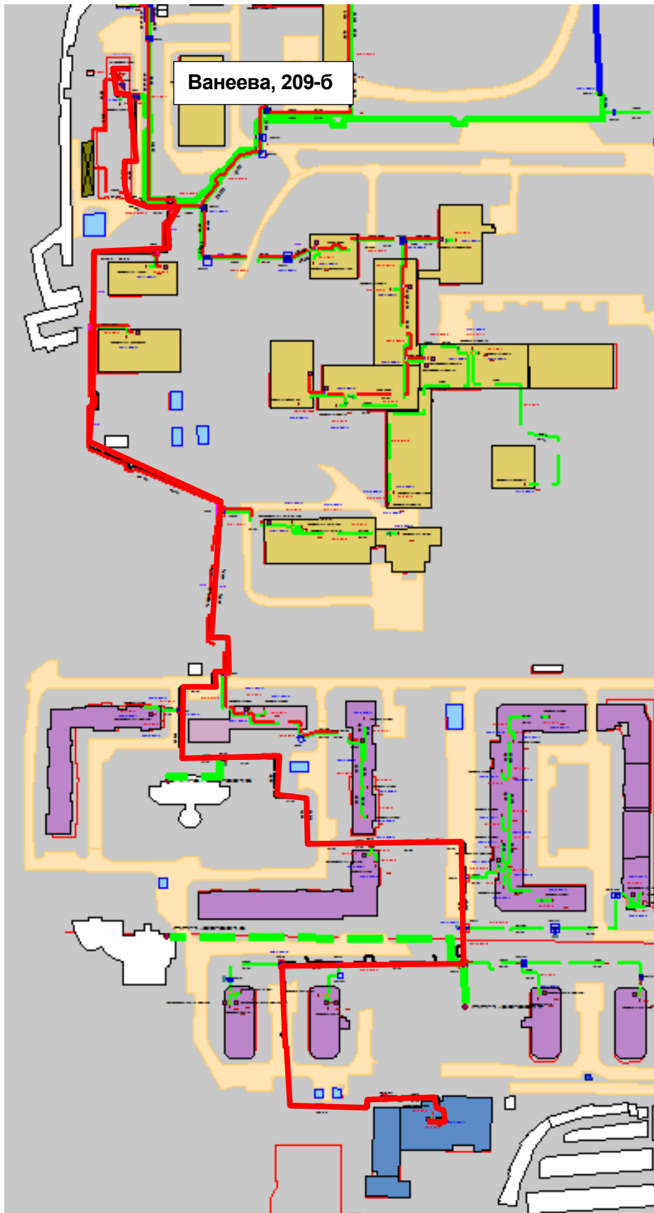
Рисунок Ошибка! Текст указанного стиля в документе отсутствует..175 – Результат гидравлического расчета - расчетный путь теплоносителя от котельной Ванеева, д.209-б до ПТ-Ванеева_Пож.депо
