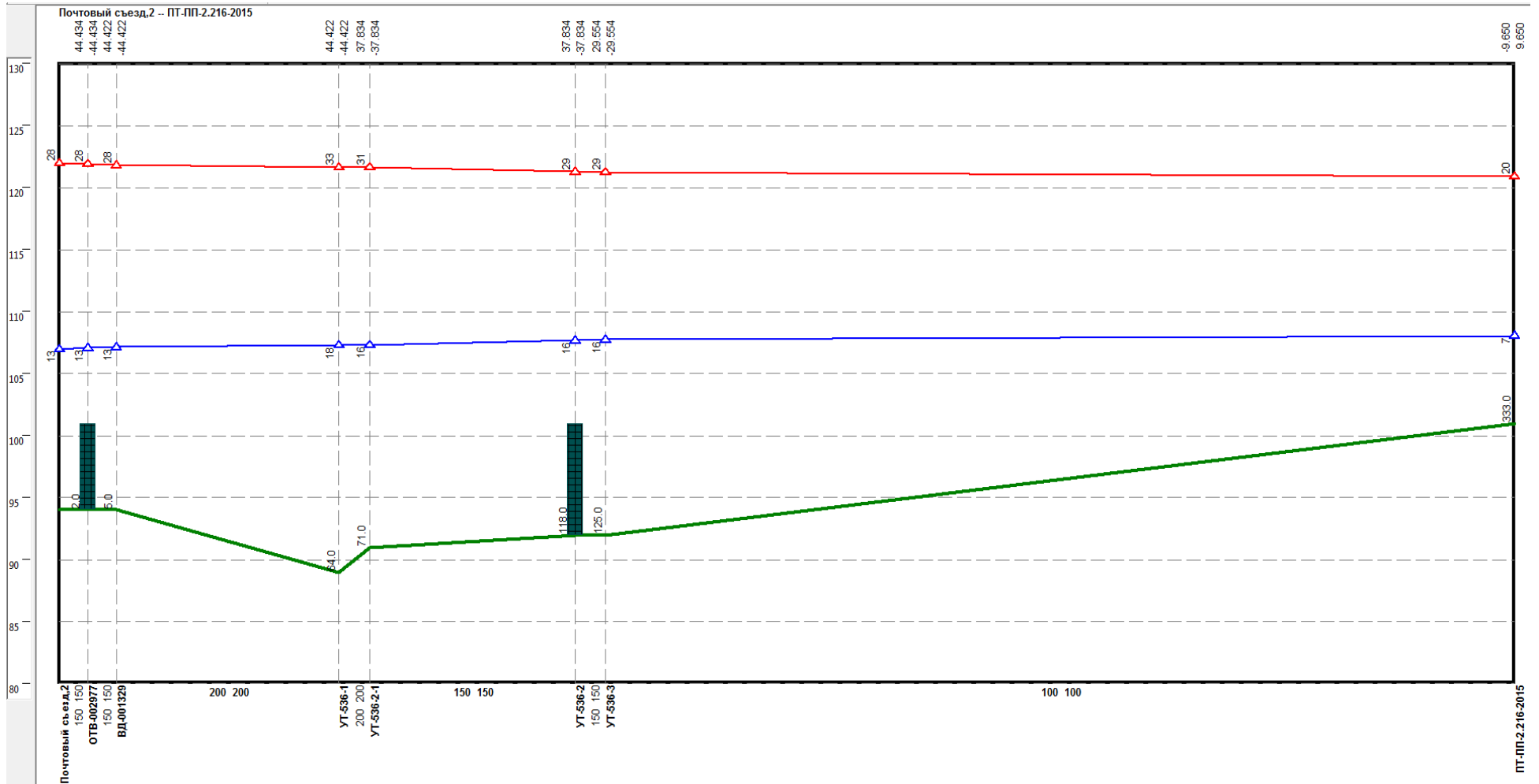
Рисунок 208 – Результат гидравлического расчета - график гидравлических режимов по пути теплоносителя от котельной Почтовый съезд, 2, 24 до ПТ-ПП-2.216-2015
