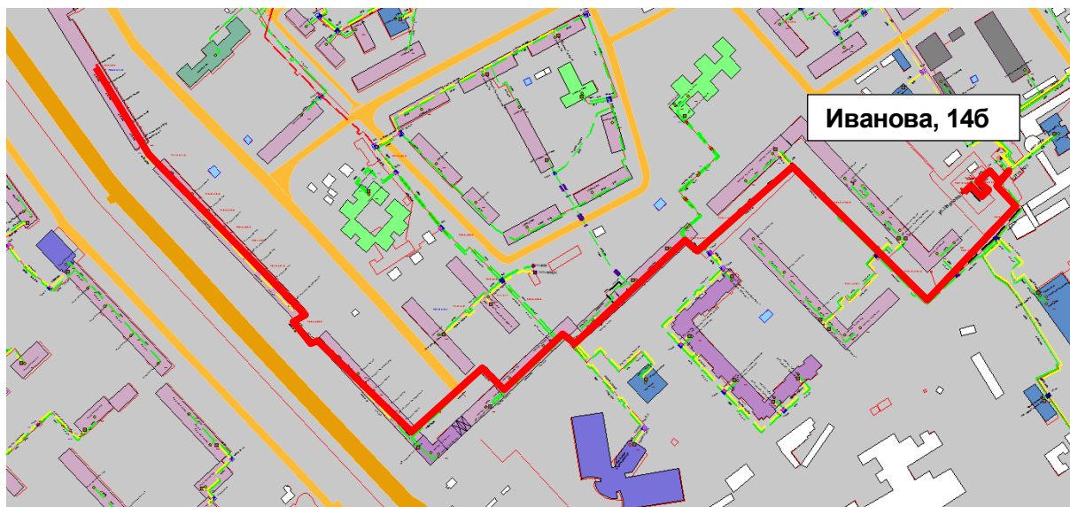
Рисунок Ошибка! Текст указанного стиля в документе отсутствует..229 – Результат гидравлического расчета - расчетный путь теплоносителя от котельной Сбербанк до ПТ-ПП-1.17-2017-2022
