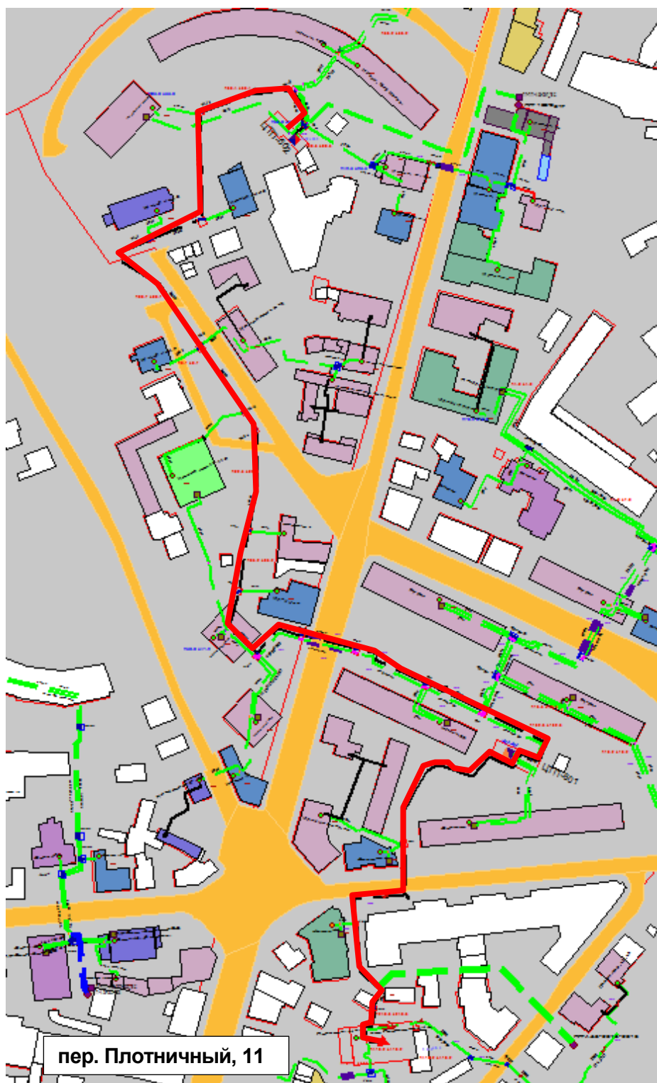
Рисунок Ошибка! Текст указанного стиля в документе отсутствует.185 – Результат гидравлического расчета - расчетный путь теплоносителя от котельной пер. Плотничный, 11 до ЦТП-602
