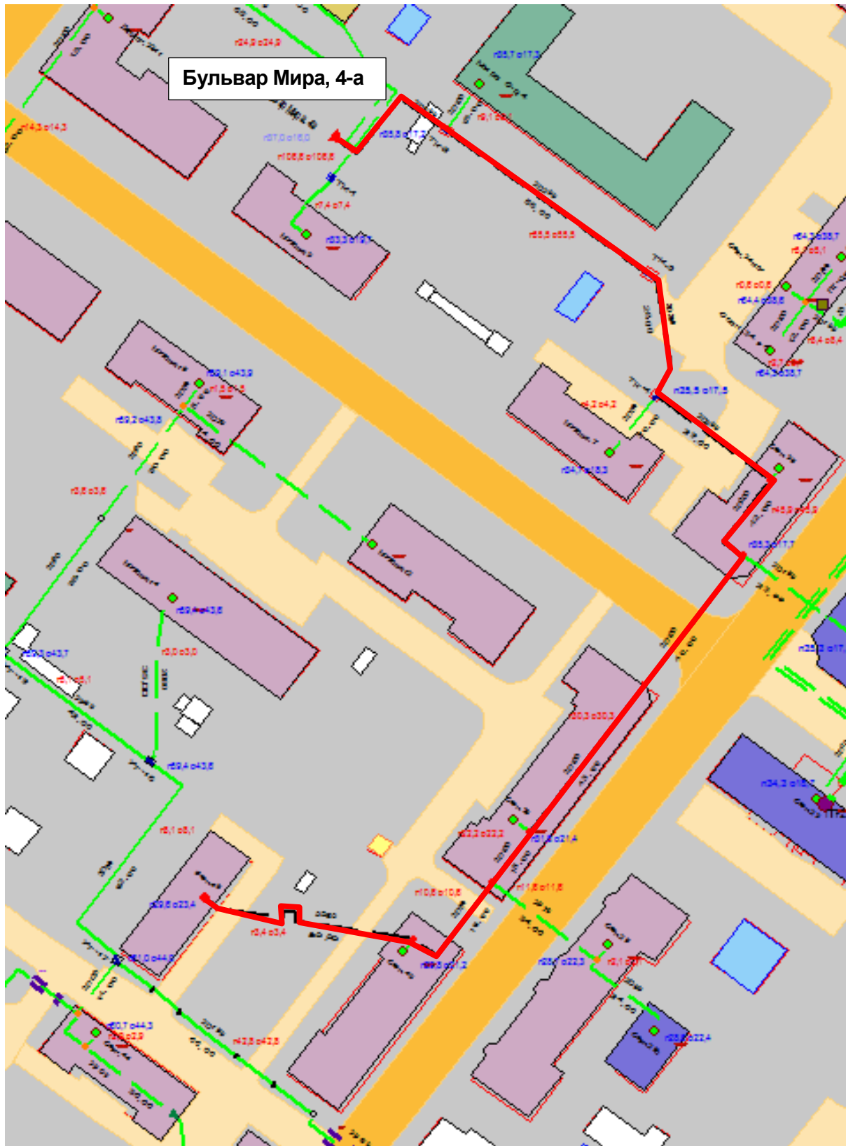
Рисунок Ошибка! Текст указанного стиля в документе отсутствует..171 – Результат гидравлического расчета - расчетный путь теплоносителя от котельной Бульвар Мира, 4-а до ПТ-Совн,46
