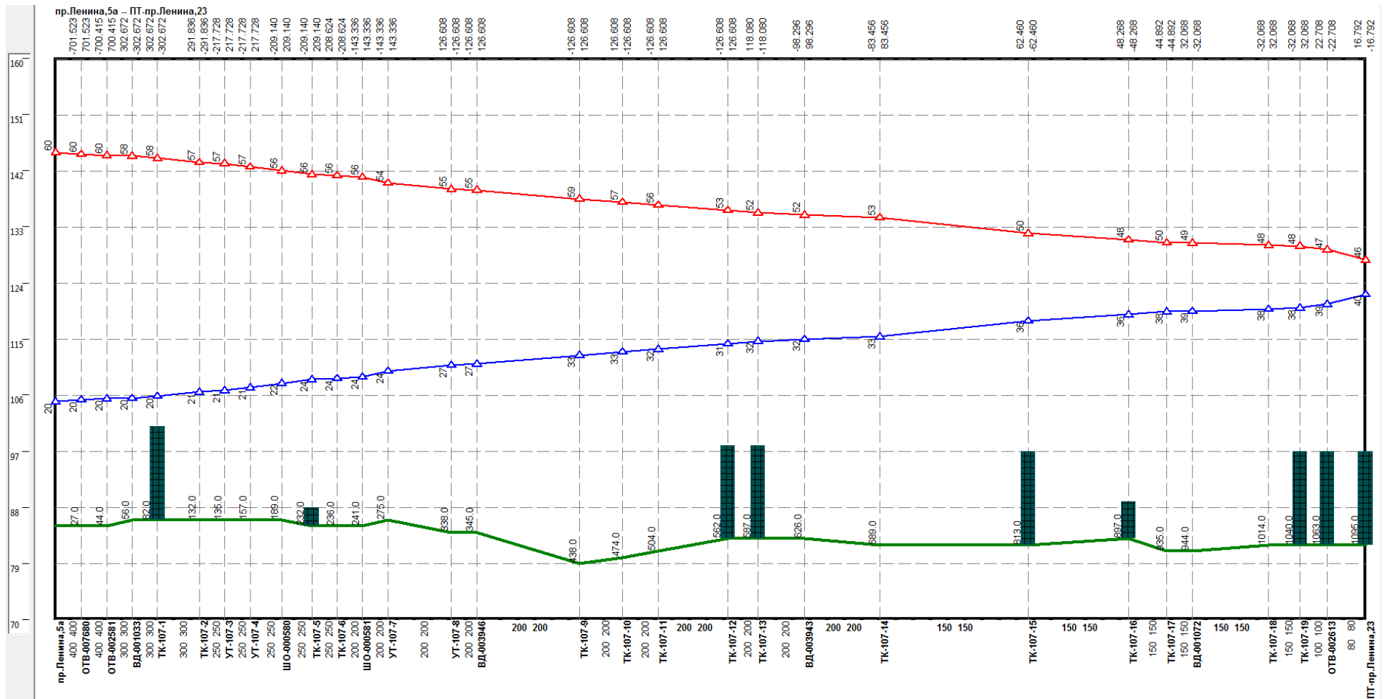
Рисунок Ошибка! Текст указанного стиля в документе отсутствует..190 –Результат гидравлического расчета - график гидравлических режимов по пути теплоносителя от котельной пр. Ленина, 5-а до ПТ-пр.Ленина,23
