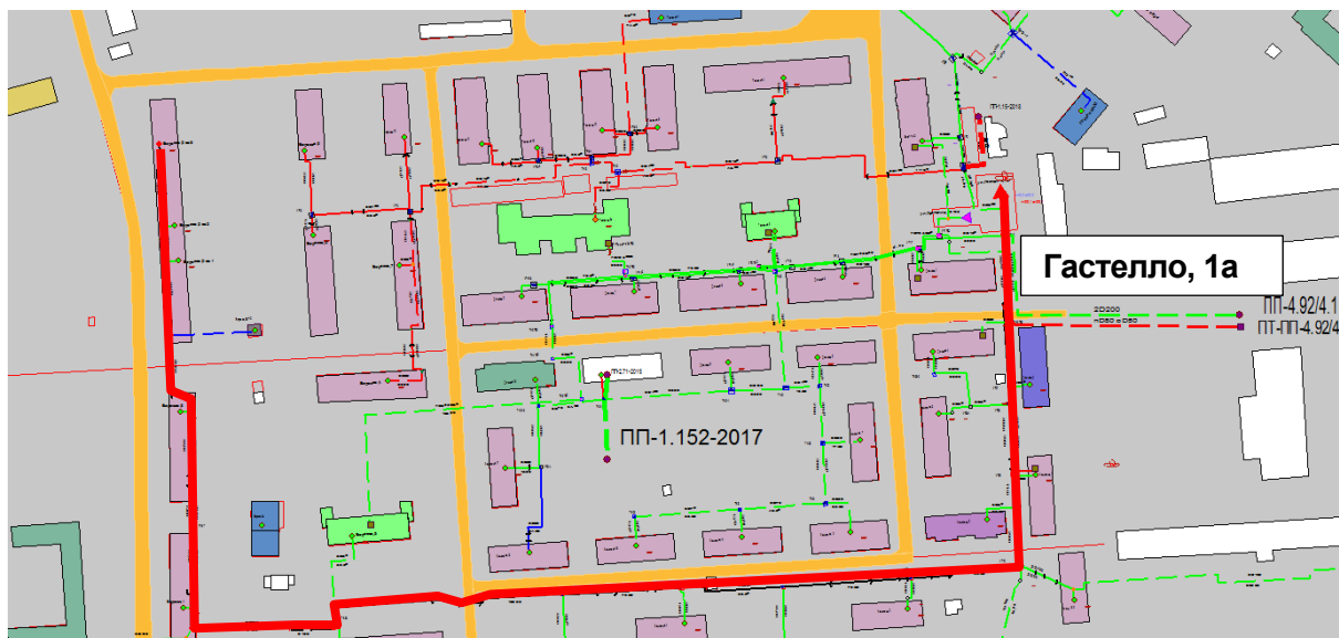
Рисунок 1.9 – Результат гидравлического расчета - расчетный путь теплоносителя от котельной Гастелло, д. 1а до ПТ-Березов,5 вв3
