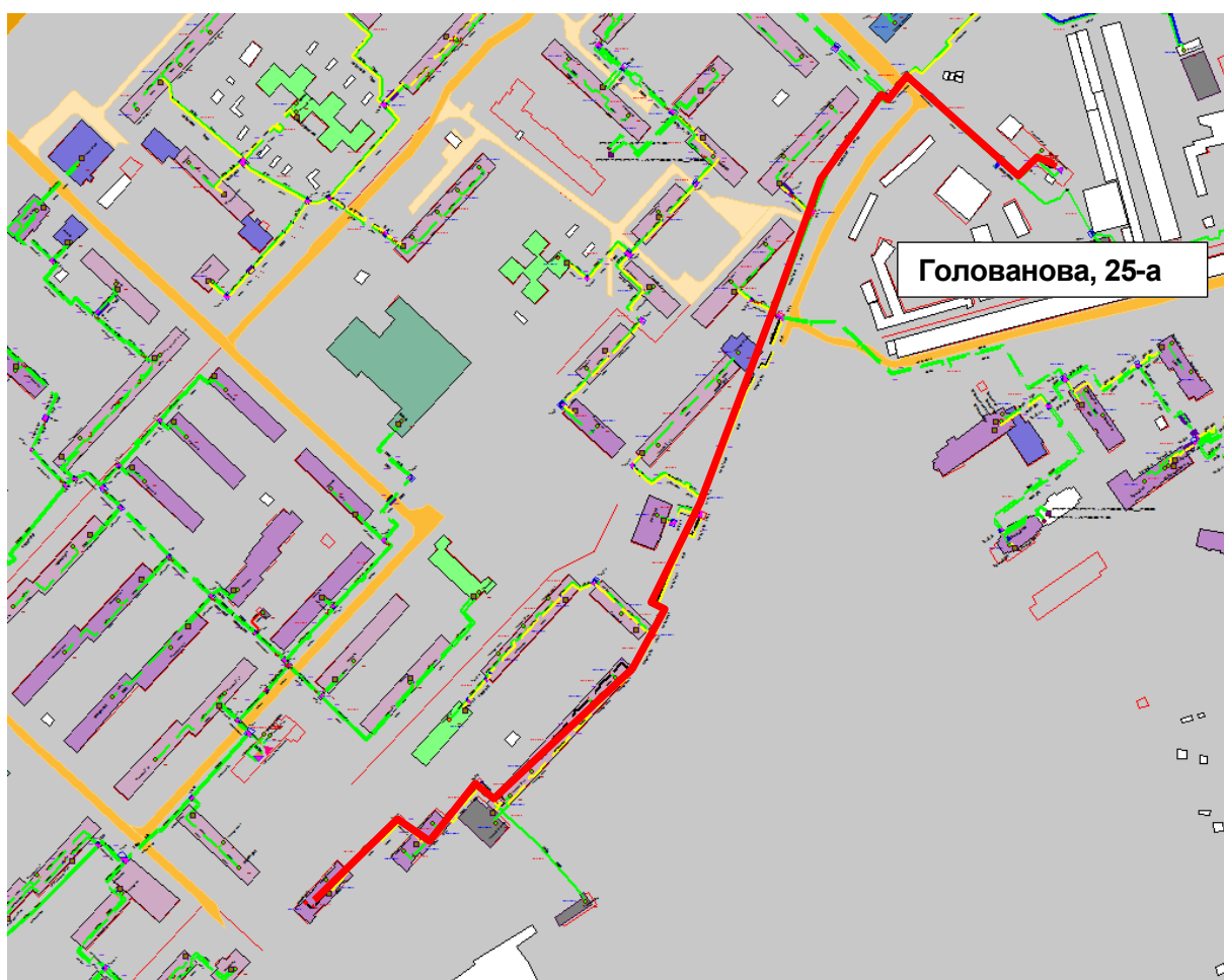
Рисунок Ошибка! Текст указанного стиля в документе отсутствует..219 – Результат гидравлического расчета - расчетный путь теплоносителя от котельной Голованова, 25-а до ПТ-Голован,57 э2
