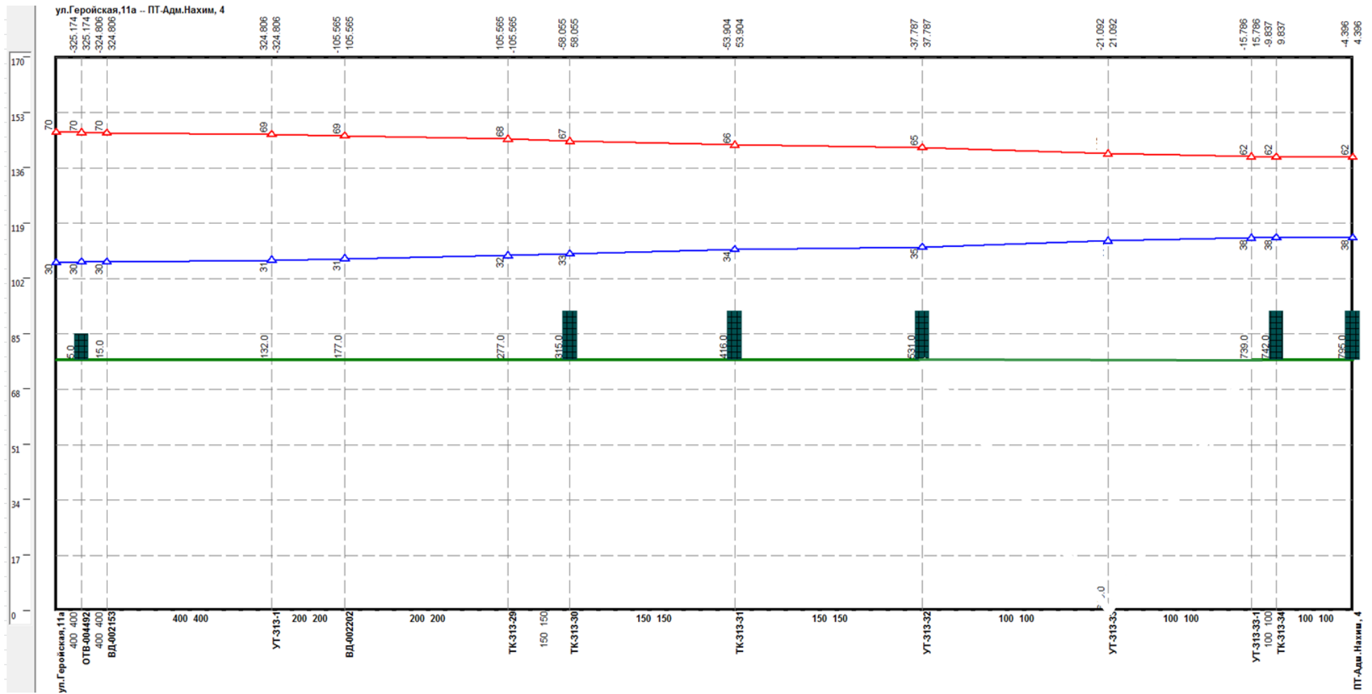
Рисунок Ошибка! Текст указанного стиля в документе отсутствует..162 –Результат гидравлического расчета - график гидравлических режимов по пути теплоносителя от котельной Геройская, 11а до ПТ-Адм.Нахим, 4
