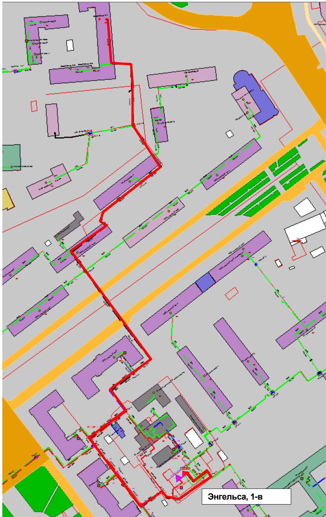
Рисунок Ошибка! Текст указанного стиля в документе отсутствует..197 – Результат гидравлического расчета - расчетный путь теплоносителя от котельной Энгельса, 1-в до ПТ-Ефрем,2 з1
