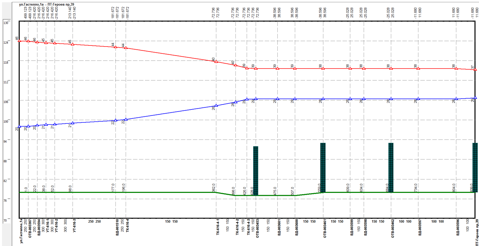
Рисунок Ошибка! Текст указанного стиля в документе отсутствует. 154 –Результат гидравлического расчета - график гидравлических режимов по пути теплоносителя от котельной Гастелло, 1а до ПТ-Героев пр,39
