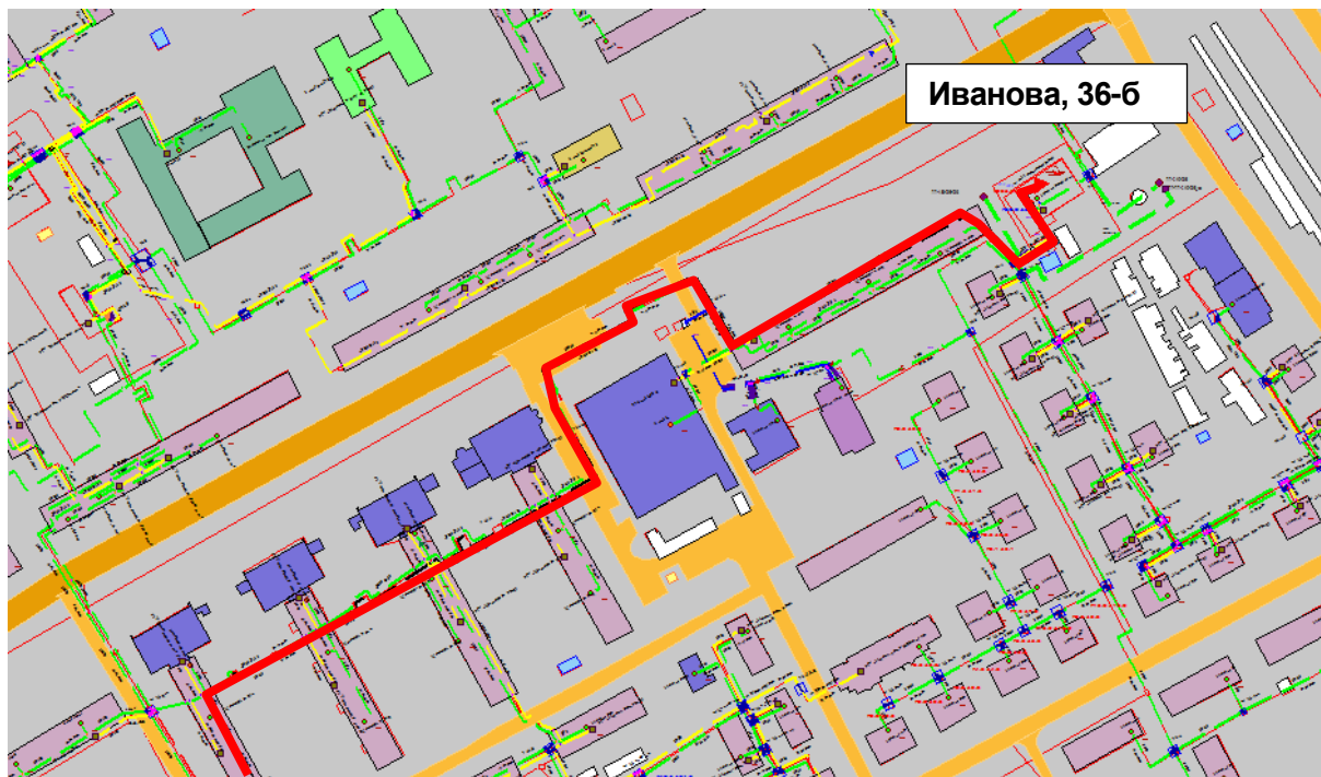
Рисунок Ошибка! Текст указанного стиля в документе отсутствует..215 – Результат гидравлического расчета - расчетный путь теплоносителя от котельной Иванова, 36-б до ПТ-Кораб,9 Э2
