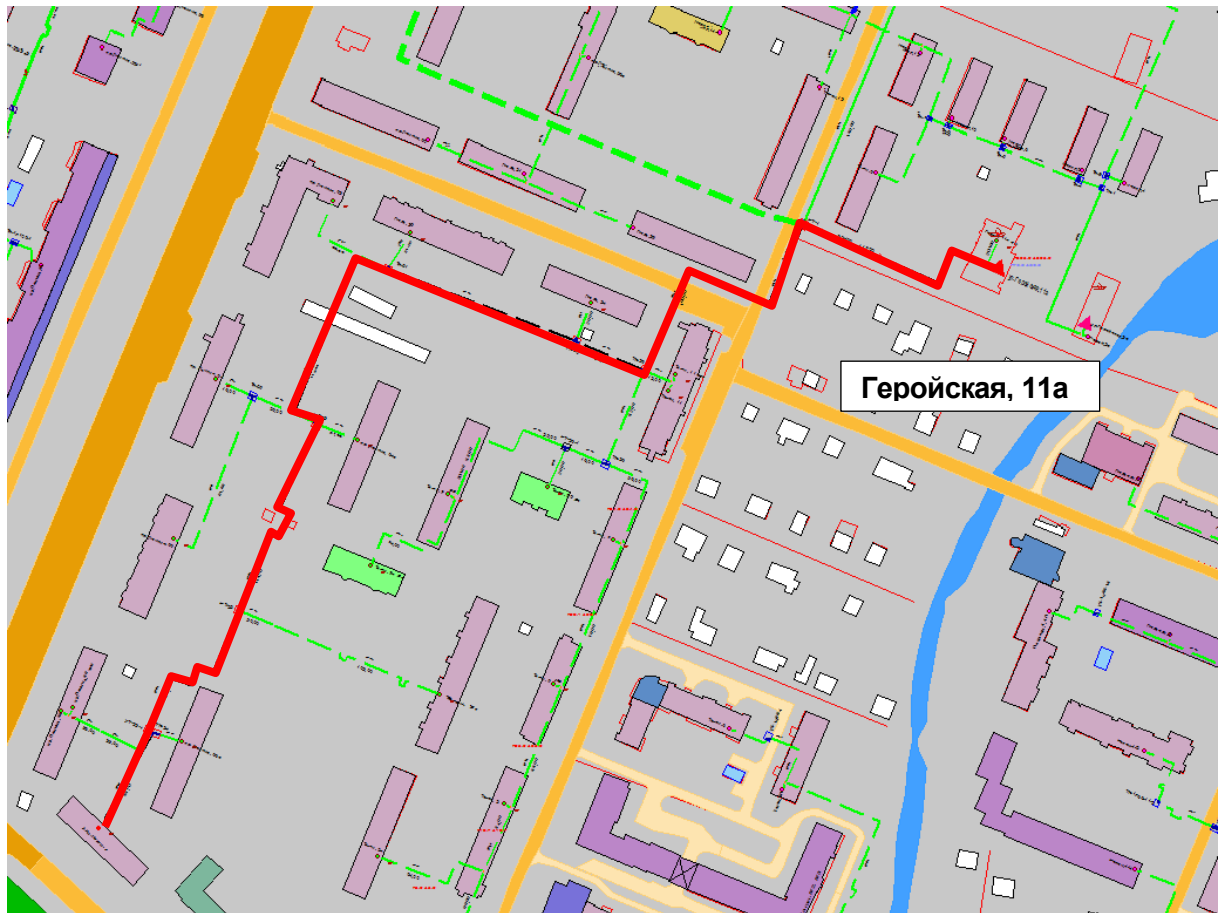
Рисунок Ошибка! Текст указанного стиля в документе отсутствует..161 – Результат гидравлического расчета - расчетный путь теплоносителя от котельной Геройская, 11а до ПТ-Адм.Нахим, 4
