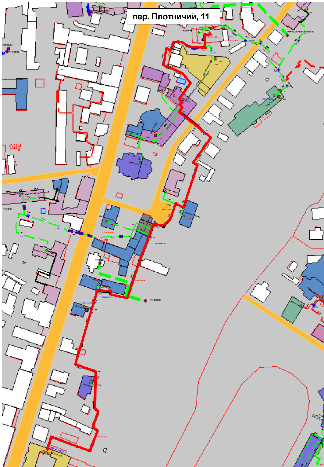
Рисунок Ошибка! Текст указанного стиля в документе отсутствует..183 – Результат гидравлического расчета - расчетный путь теплоносителя от котельной пер. Плотничий, 11 до ПТ-Ильин,78,78а,гар
