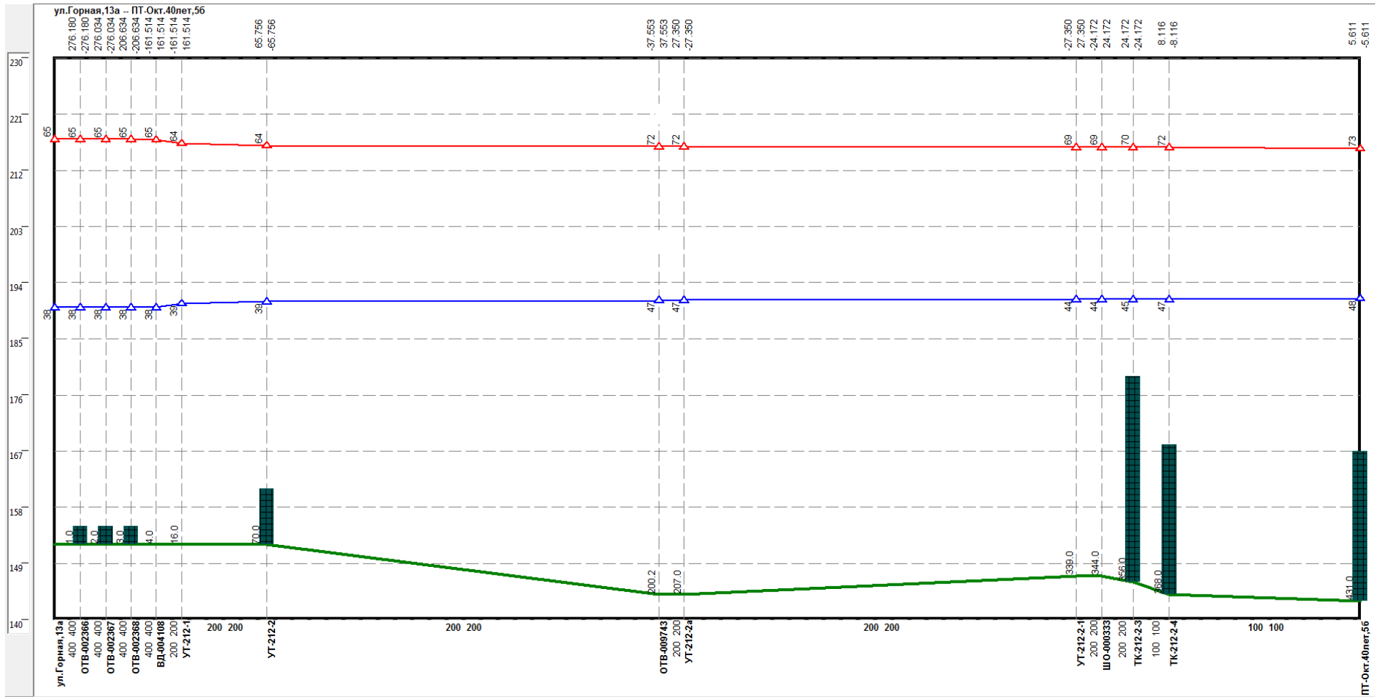
Рисунок Ошибка! Текст указанного стиля в документе отсутствует.182 –Результат гидравлического расчета - график гидравлических режимов по пути теплоносителя 2 от котельной Горная, 13-а до ПТ-Окт.40лет,56
