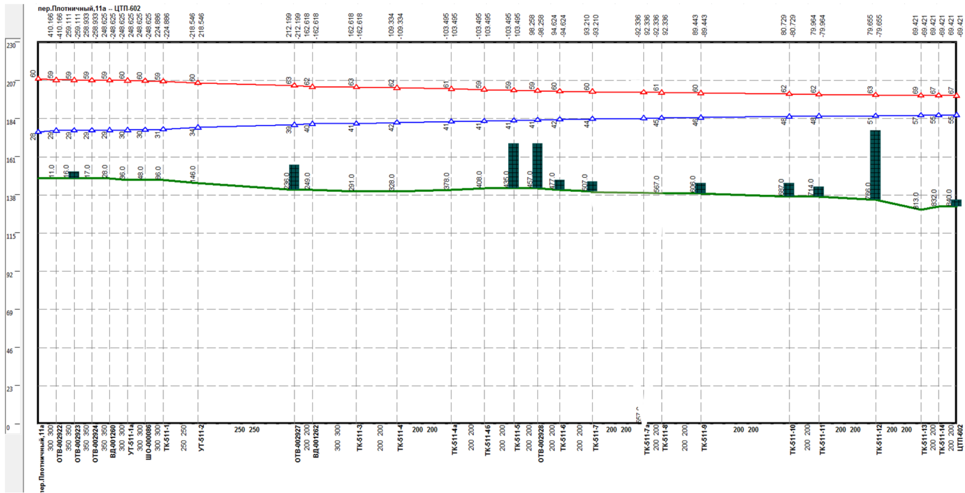
Рисунок Ошибка! Текст указанного стиля в документе отсутствует..186 –Результат гидравлического расчета - график гидравлических режимов по пути теплоносителя от котельной пер. Плотничный, 11 до ЦТП-602
