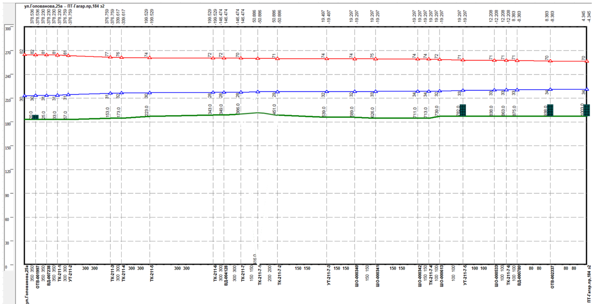
Рисунок Ошибка! Текст указанного стиля в документе отсутствует..218 –Результат гидравлического расчета - график гидравлических режимов по пути теплоносителя от котельной Голованова, 25-а до ПТ-Гагар.пр,184 э2
