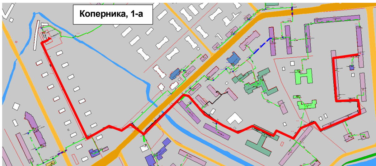
Рисунок Ошибка! Текст указанного стиля в документе отсутствует.223 – Результат гидравлического расчета - расчетный путь теплоносителя от котельной Коперника, 1-а до ПТ-Рыбак, 10/1
