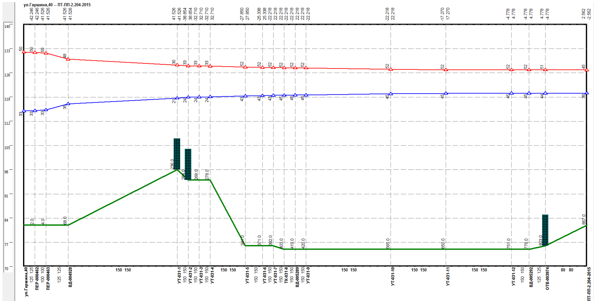
Рисунок Ошибка! Текст указанного стиля в документе отсутствует..160 –Результат гидравлического расчета - график гидравлических режимов по пути теплоносителя от котельной ООО «НКХП-Девелопмент» до ПТ-ПН-2.204-2015
