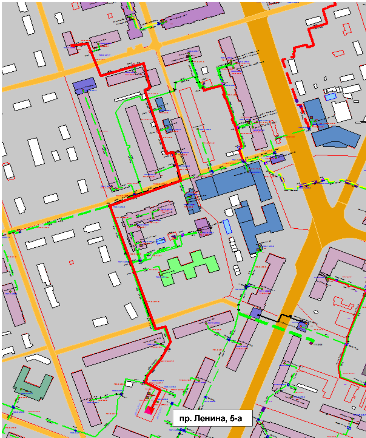
Рисунок Ошибка! Текст указанного стиля в документе отсутствует..191 – Результат гидравлического расчета - расчетный путь теплоносителя от котельной пр. Ленина, 5-а до ПТ-Чонгар,22
