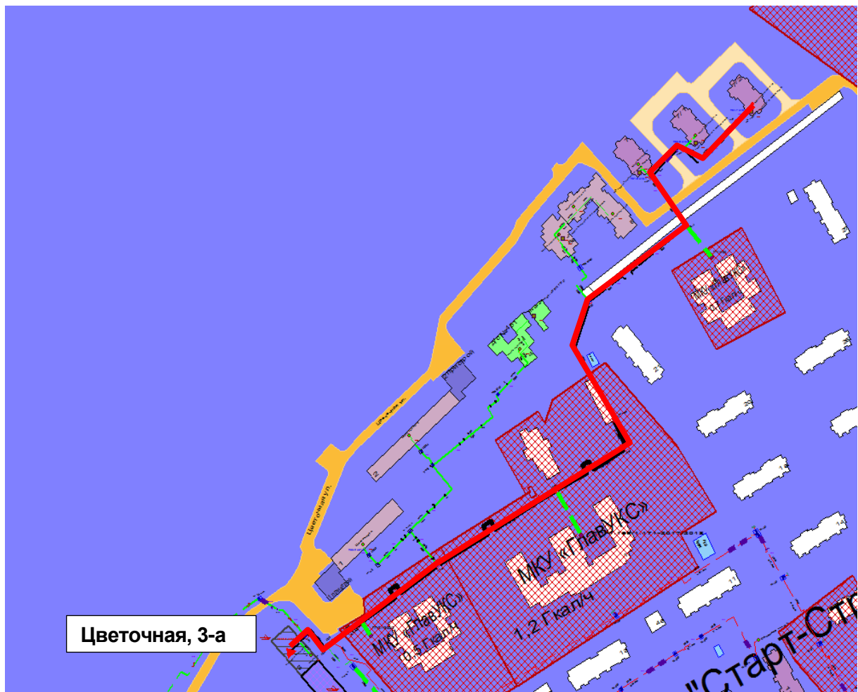
Рисунок Ошибка! Текст указанного стиля в документе отсутствует..225 – Результат гидравлического расчета - расчетный путь теплоносителя от котельной Цветочная, 3-а до ПТ-Цветочная,7/2
