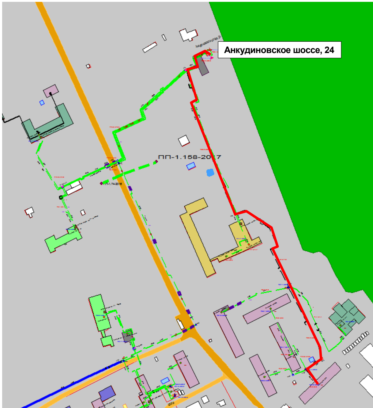
Рисунок Ошибка! Текст указанного стиля в документе отсутствует..193 – Результат гидравлического расчета - расчетный путь теплоносителя от котельной Анкудиновское шоссе, 24 до ПТ-Анкуд.ш,30
