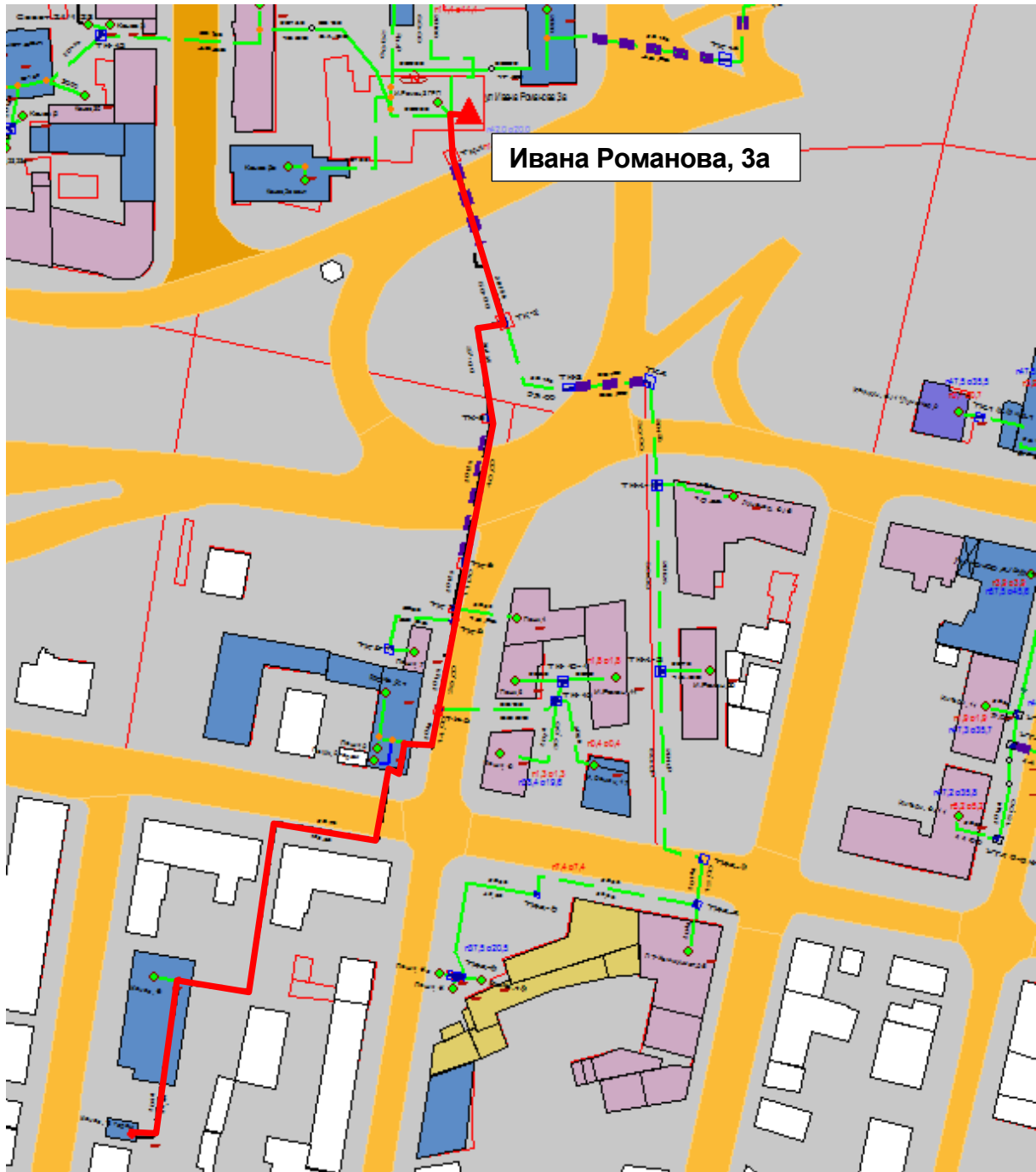
Рисунок Ошибка! Текст указанного стиля в документе отсутствует..145 - Результат гидравлического расчета - расчетный путь теплоносителя от котельной Ивана Романова, 3а до ПТ-Канав, 16 гараж
