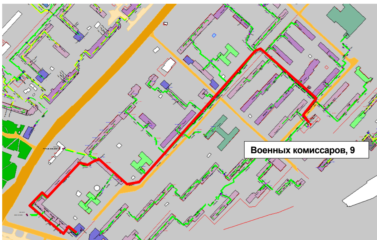
Рисунок Ошибка! Текст указанного стиля в документе отсутствует..205 – Результат гидравлического расчета - расчетный путь теплоносителя от от котельной Военных комиссаров, 9 до ПТ-Гагар.пр,226 пристр
