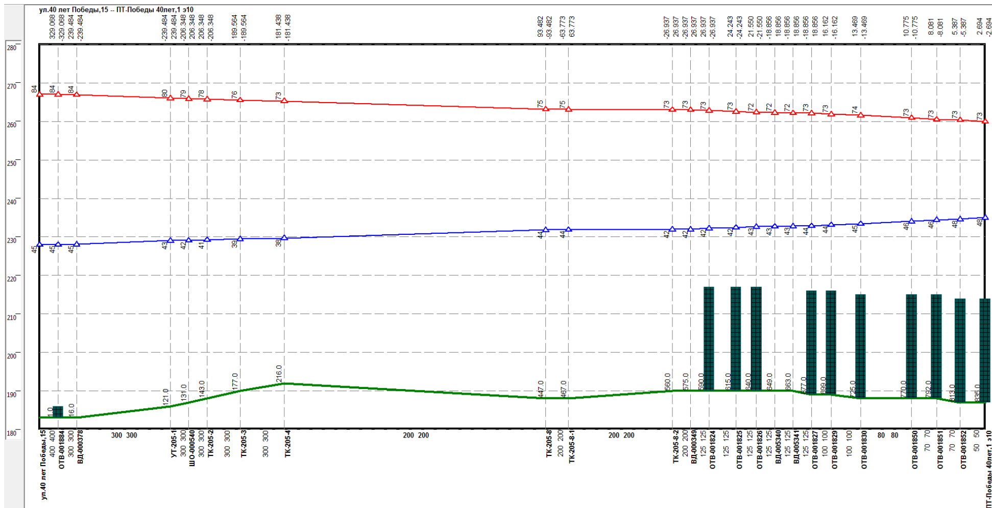
Рисунок Ошибка! Текст указанного стиля в документе отсутствует...204 –Результат гидравлического расчета - график гидравлических режимов по пути теплоносителя от котельной 40 лет Победы, д.15 до ПТ-Победы 40лет,1 э10
