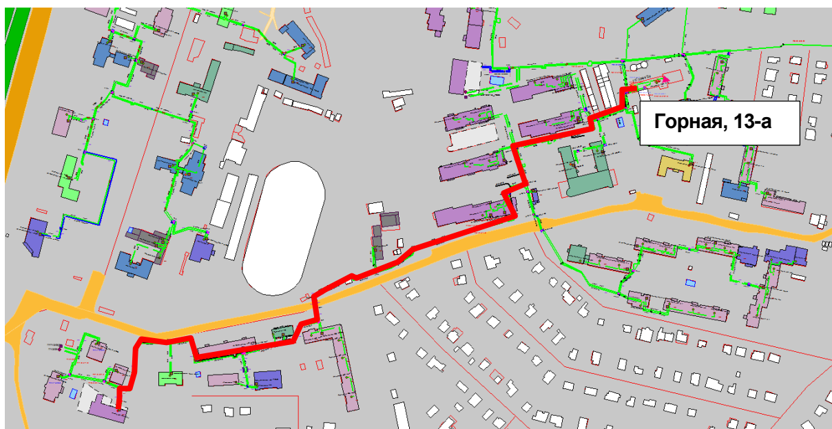
Рисунок Ошибка! Текст указанного стиля в документе отсутствует..179 – Результат гидравлического расчета - расчетный путь теплоносителя от котельной Горная, 13-а до ПТ-Горная,2(стр.)
