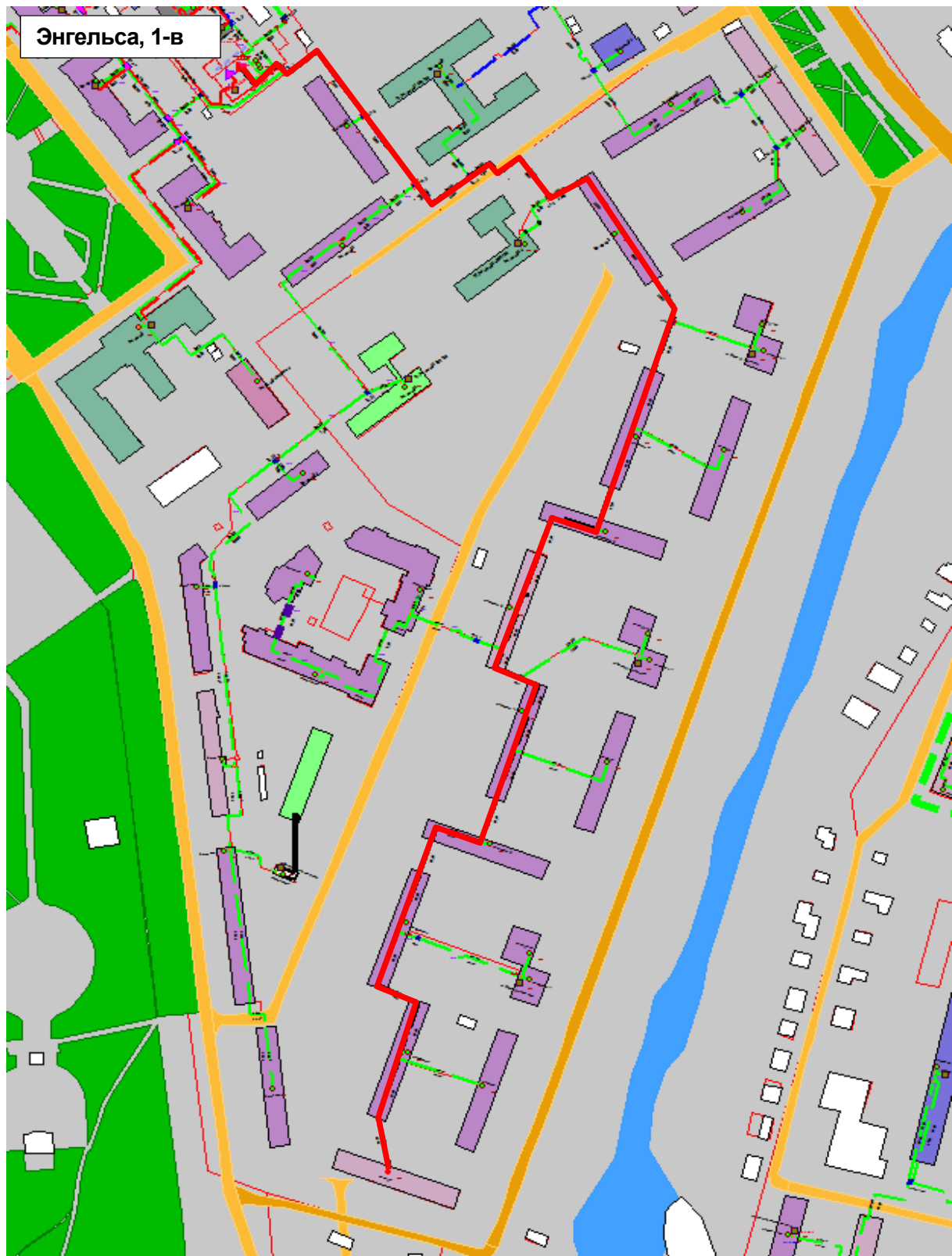
Рисунок Ошибка! Текст указанного стиля в документе отсутствует..201 – Результат гидравлического расчета - расчетный путь теплоносителя от котельной Энгельса, 1-в до ПТ-Больш,7
