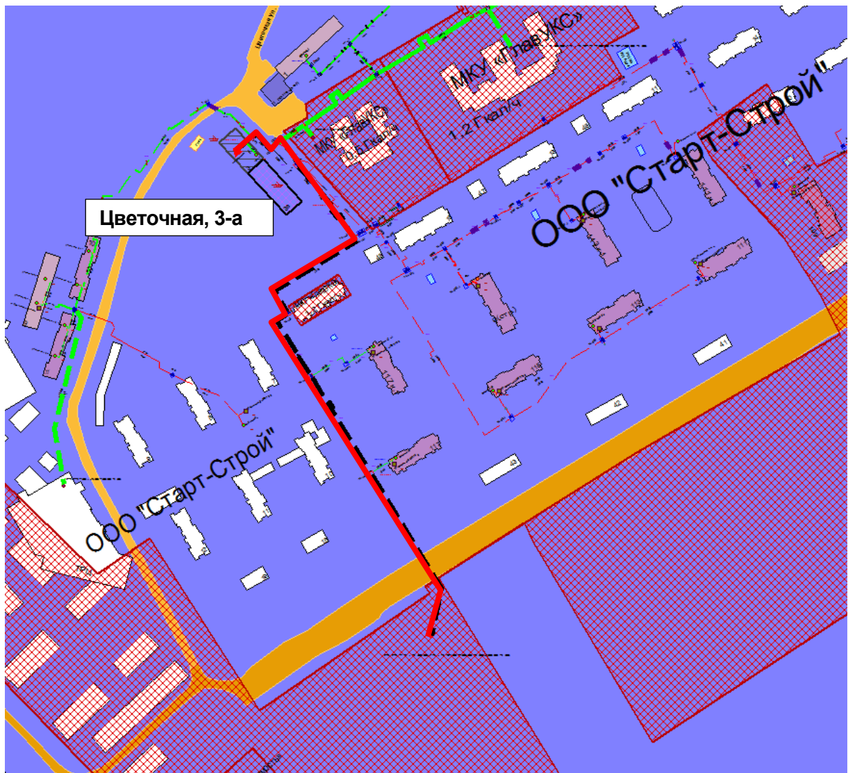
Рисунок Ошибка! Текст указанного стиля в документе отсутствует..227 – Результат гидравлического расчета - расчетный путь теплоносителя от котельной Цветочная, 3-а до ПТ-Гаугеля,1 до ПТ-ПП-1.150/1.170-2016/2018
