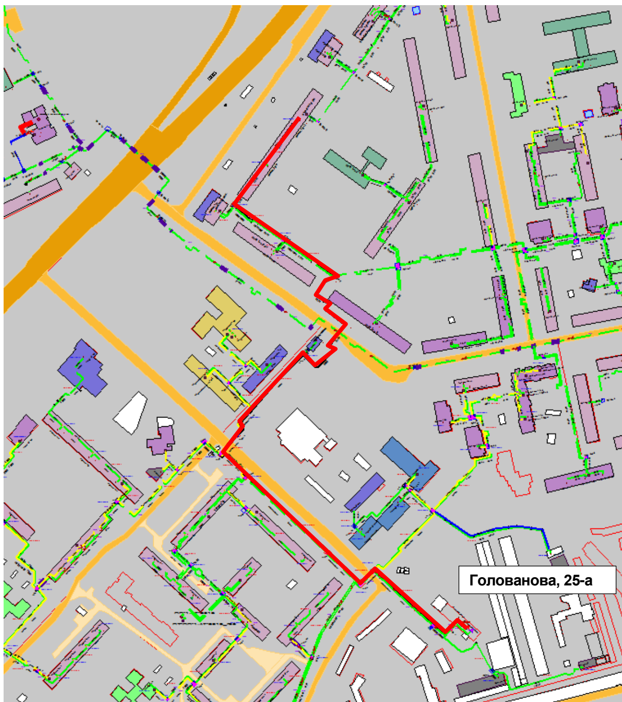
Рисунок Ошибка! Текст указанного стиля в документе отсутствует..217 – Результат гидравлического расчета - расчетный путь теплоносителя от котельной Голованова, 25-а до ПТ-Гагар.пр,184 э2
