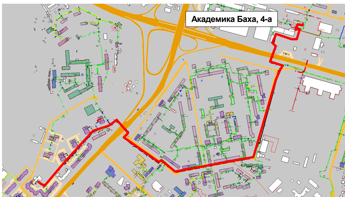
Рисунок Ошибка! Текст указанного стиля в документе отсутствует..211 – Результат гидравлического расчета - расчетный путь теплоносителя от котельной Академика Баха, 4-а до ПТ-Макар, 18 э2
