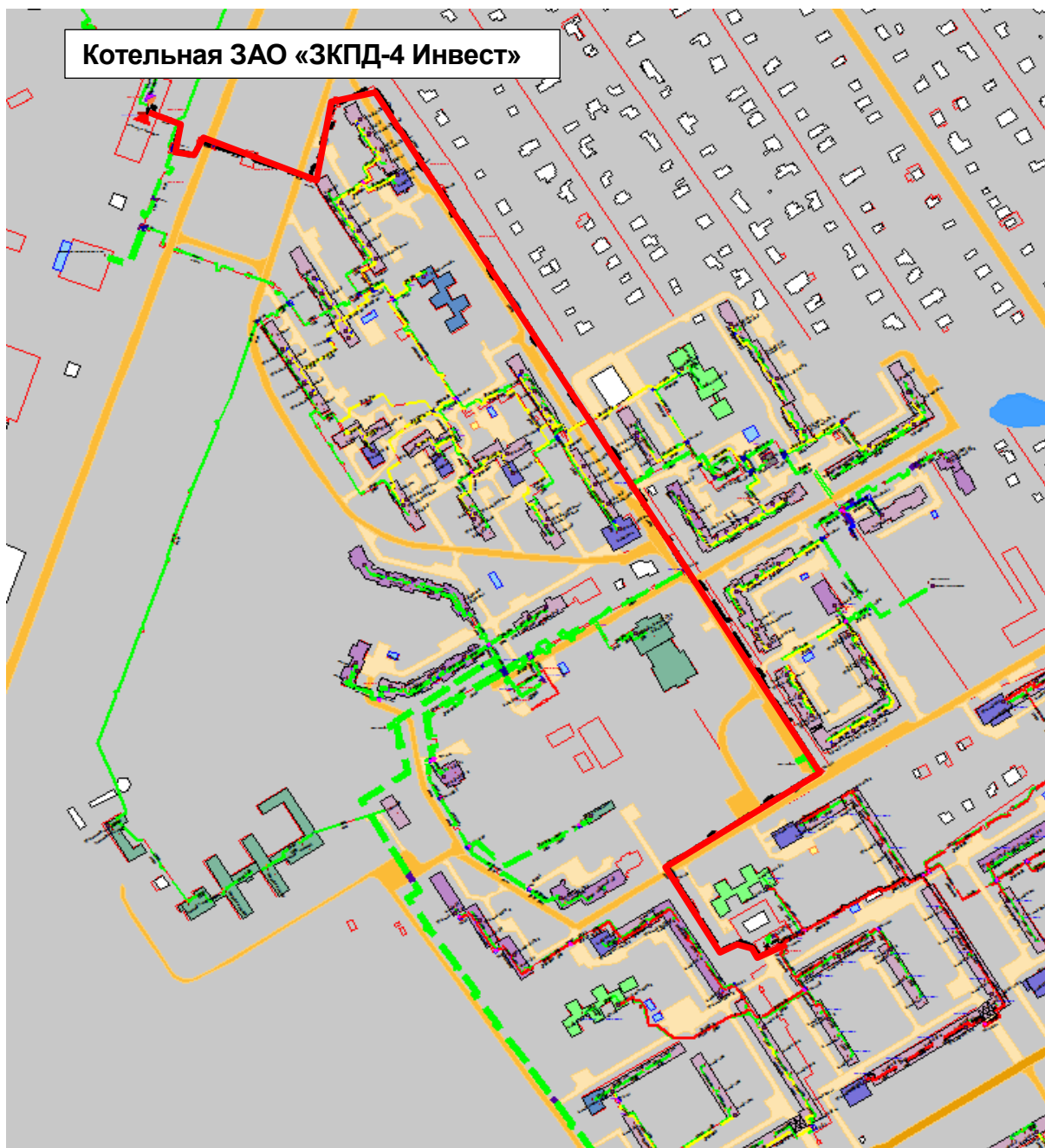
Рисунок 1.149- Результат гидравлического расчета - расчетный путь теплоносителя от котельной ЗАО «ЗКПД-4 Инвест» до ПТ-Кораб,26/2 аптека
