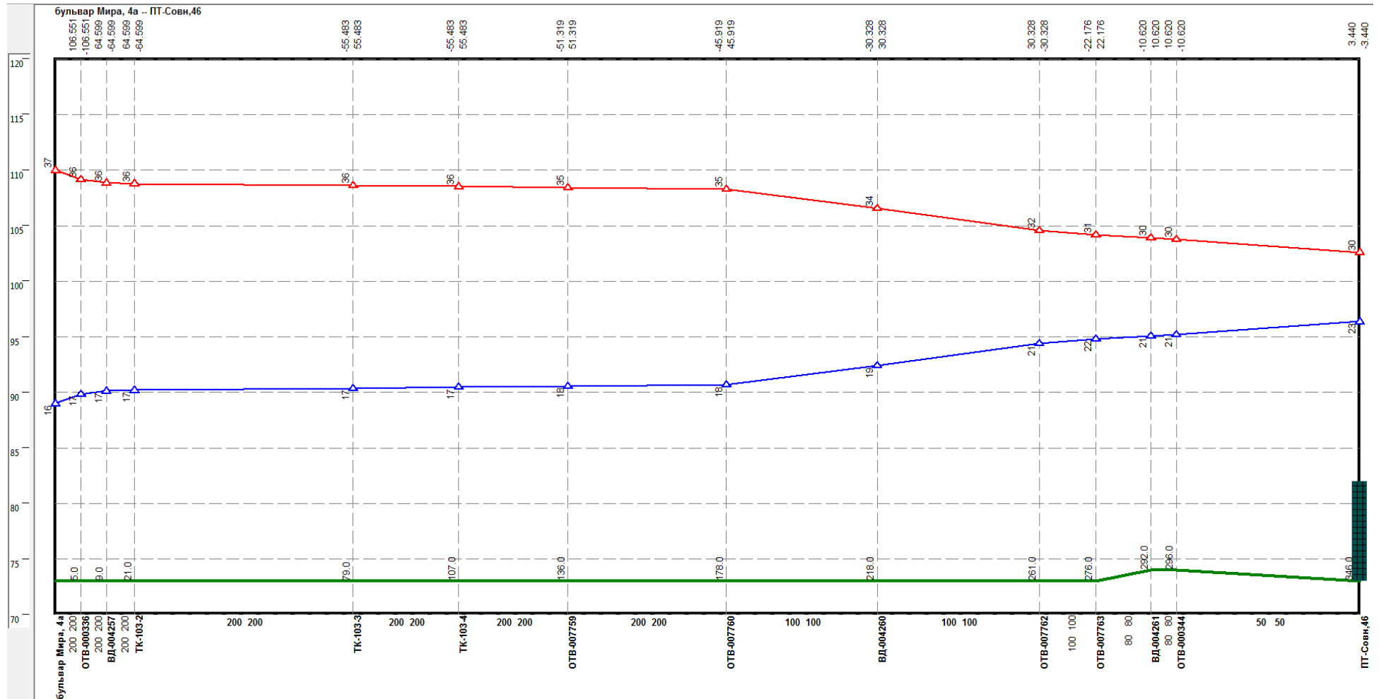
Рисунок Ошибка! Текст указанного стиля в документе отсутствует..172 –Результат гидравлического расчета - график гидравлических режимов по пути теплоносителя от котельной Бульвар Мира, 4-а до ПТ-Совн,46
