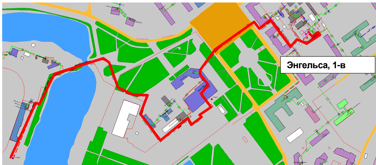
Рисунок Ошибка! Текст указанного стиля в документе отсутствует..199 – Результат гидравлического расчета - расчетный путь теплоносителя от котельной Энгельса, 1-в до ПТ-ПП-2.164-2017
