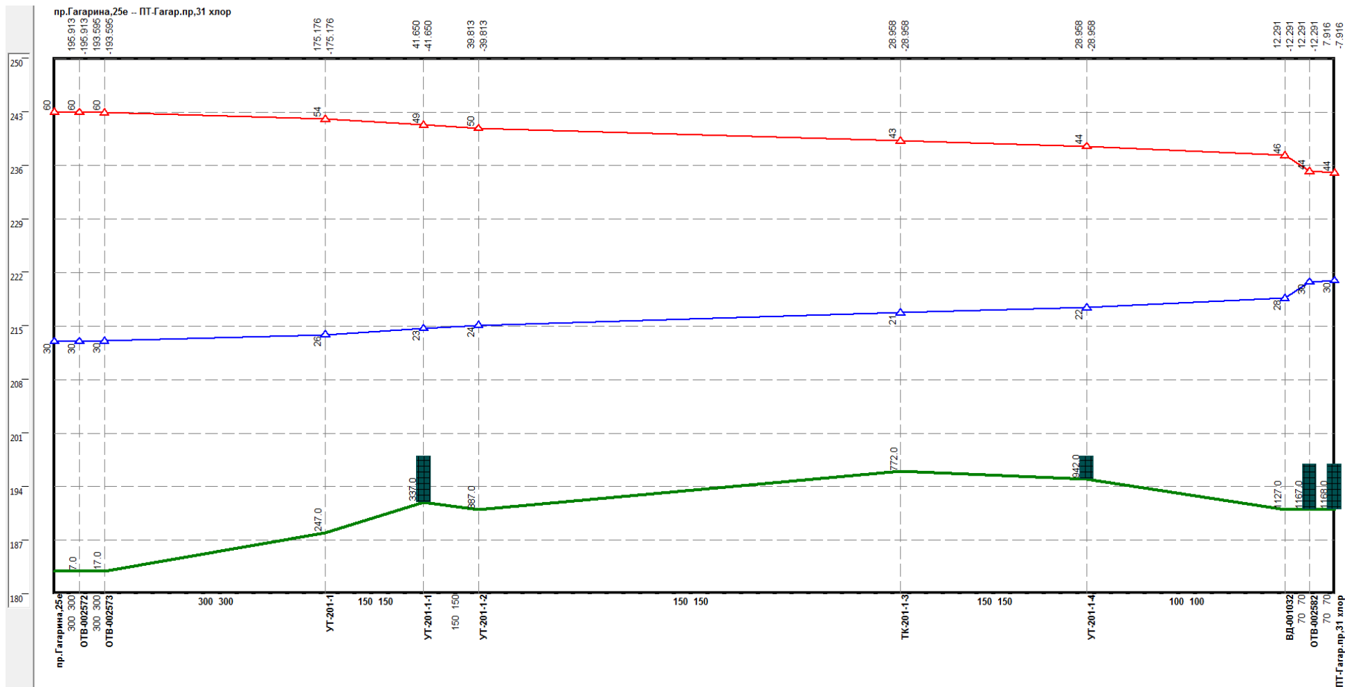
Рисунок Ошибка! Текст указанного стиля в документе отсутствует..174 –Результат гидравлического расчета - график гидравлических режимов по пути теплоносителя от котельной пр. Гагарина, 25-е до ПТ-Гагар.пр.31 хлор
