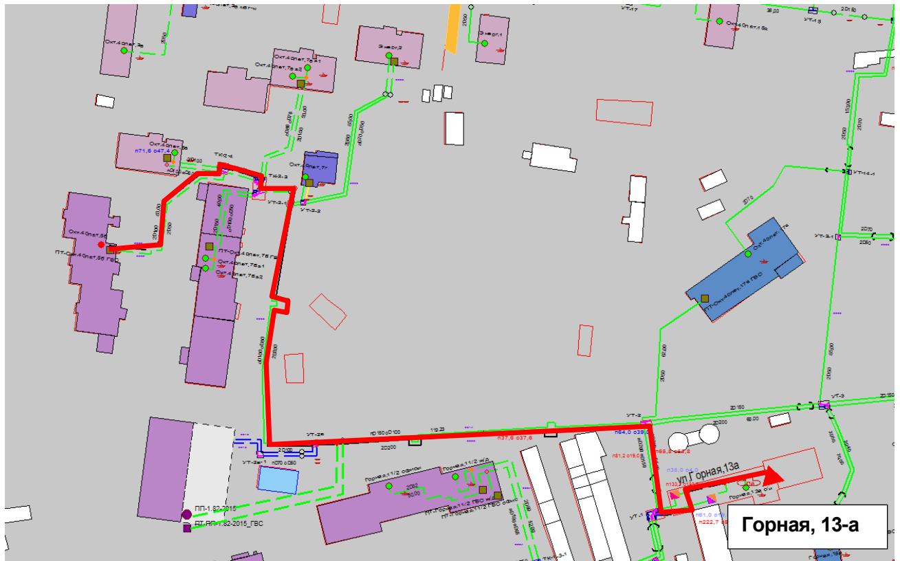
Рисунок Ошибка! Текст указанного стиля в документе отсутствует..181 – Результат гидравлического расчета - расчетный путь теплоносителя 2 от котельной Горная, 13-а до ПТ-Окт.40лет,5б
