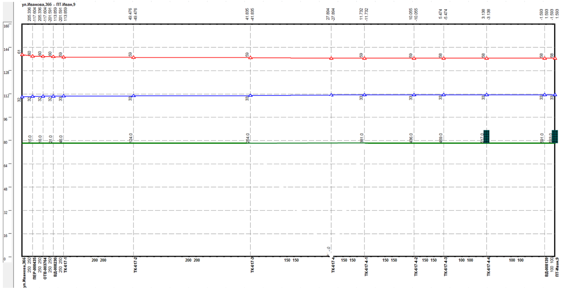
Рисунок Ошибка! Текст указанного стиля в документе отсутствует..214 –Результат гидравлического расчета - график гидравлических режимов по пути теплоносителя от котельной Иванова, 36-б до ПТ-Иван,9
