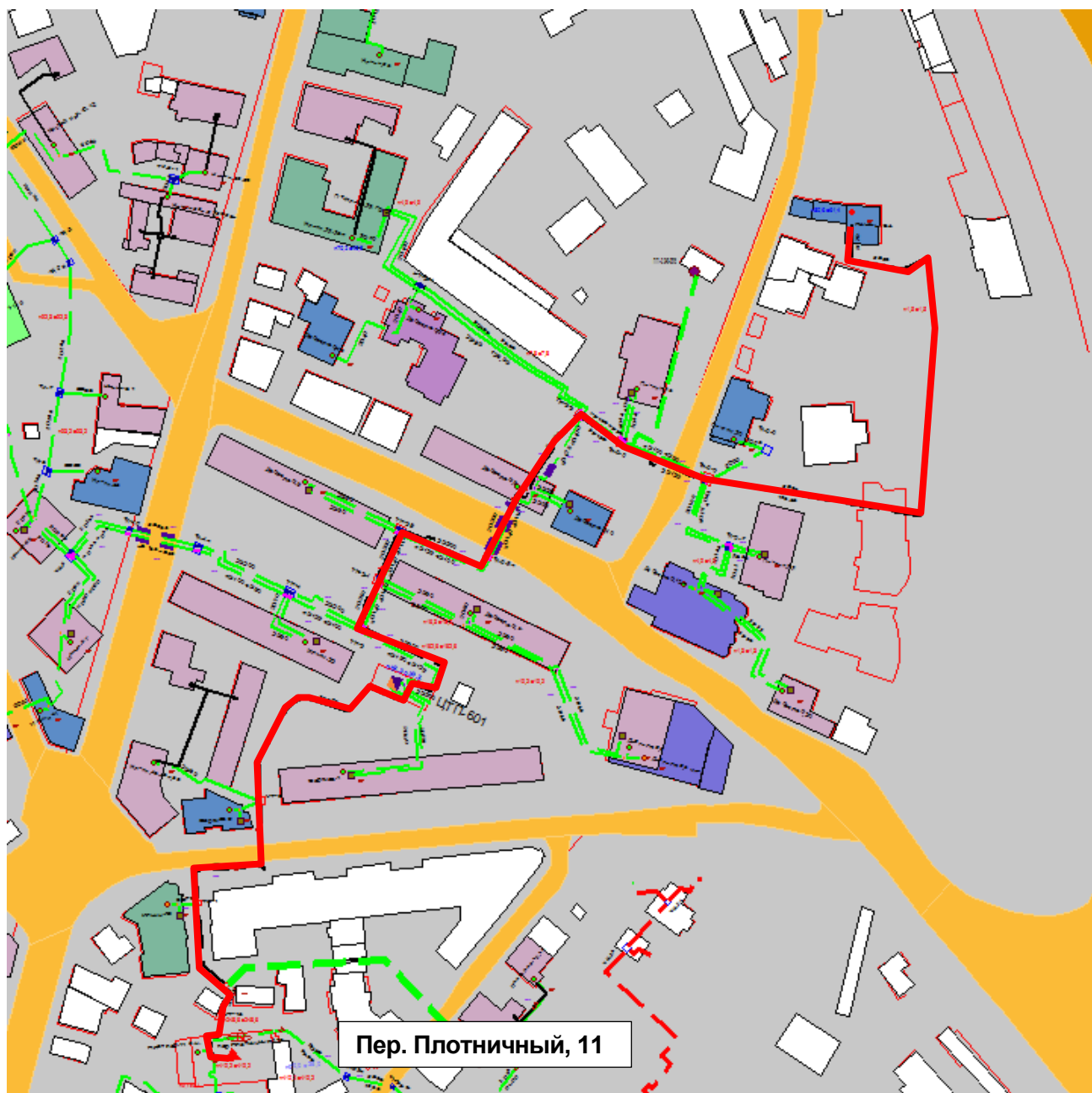
Рисунок Ошибка! Текст указанного стиля в документе отсутствует..187 – Результат гидравлического расчета - расчетный путь теплоносителя от котельной пер. Плотничный, 11 до ПТ-Почаин, 14а
